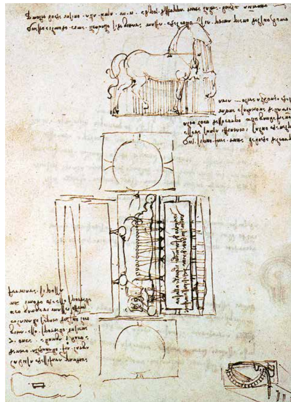
Sforců žirgo liejimo duobės eskizas, apie 1493. Šiame eskize su paaiškinamosiomis pastabomis duobė vaizduojama iš viršaus (piešinio viršuje) ir šono (apačioje).
